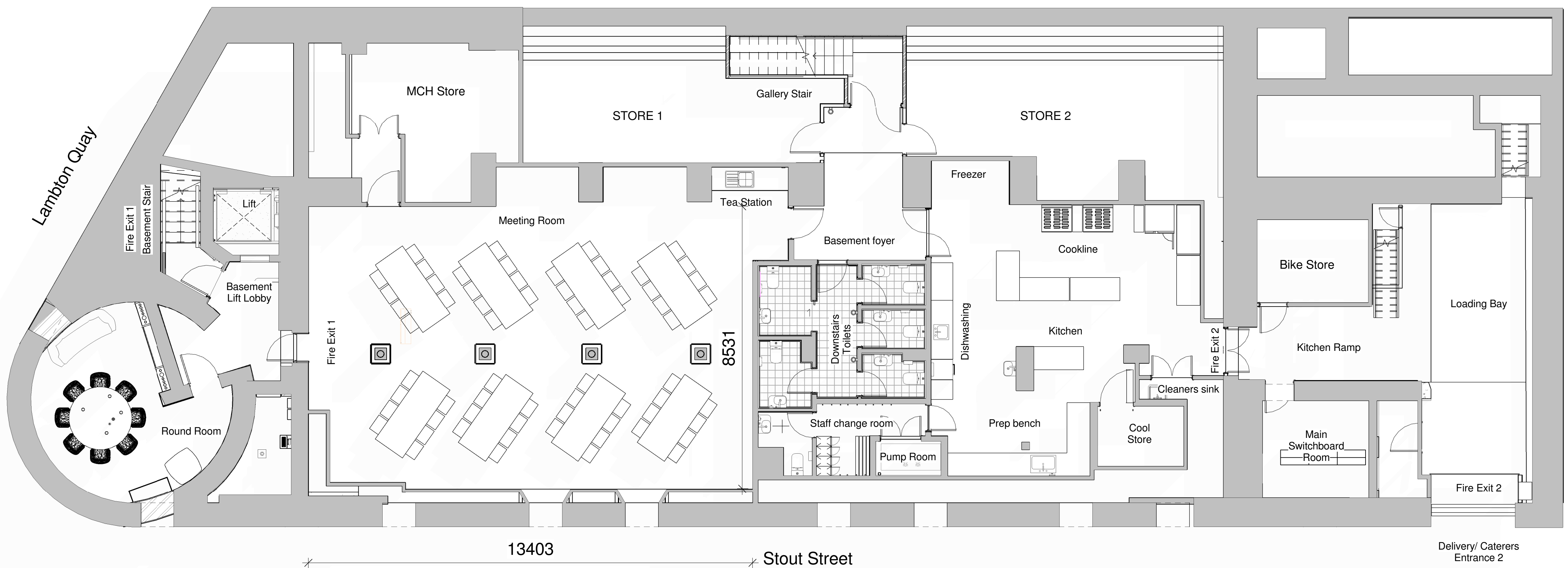
1 Basement Layout 1 : 75
